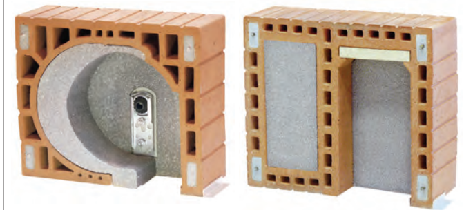
Bild 15: Ziegel-Rollladenkasten (Beispiele)
