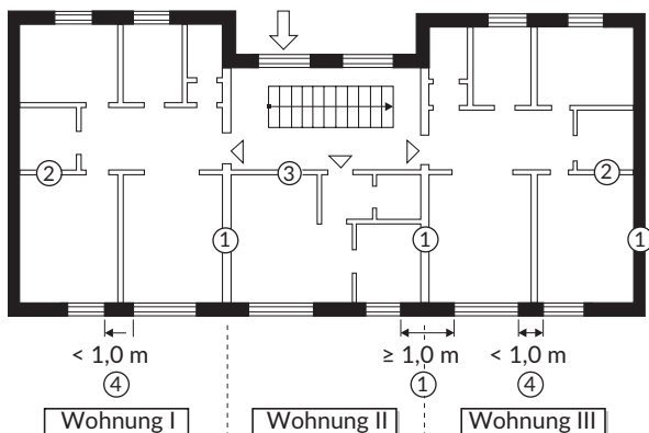
Bild 2: Benennung von Bauteilen nach DIN EN 1996-1-2/NA
